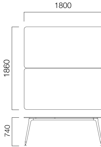
W:186 cm İkilil Masa
