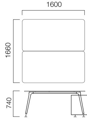
W:166 cm İkilil Üç Ayak Toplantı Masası
