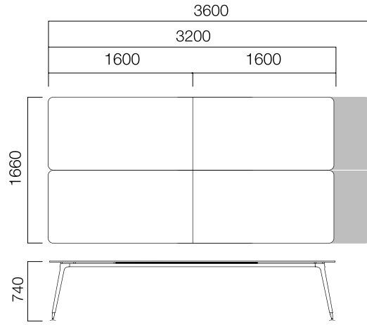
W:166 cm Dörtlü Toplantı Masası
