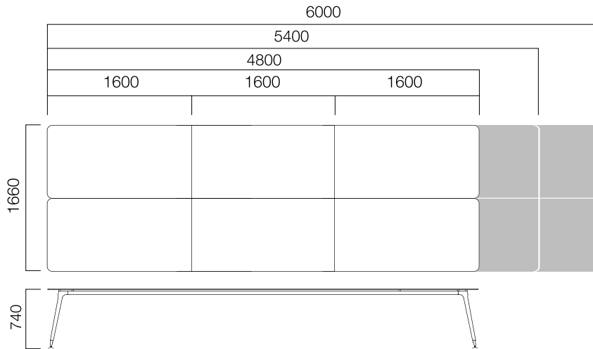
W:166 cm Altılı Toplantı Masası
