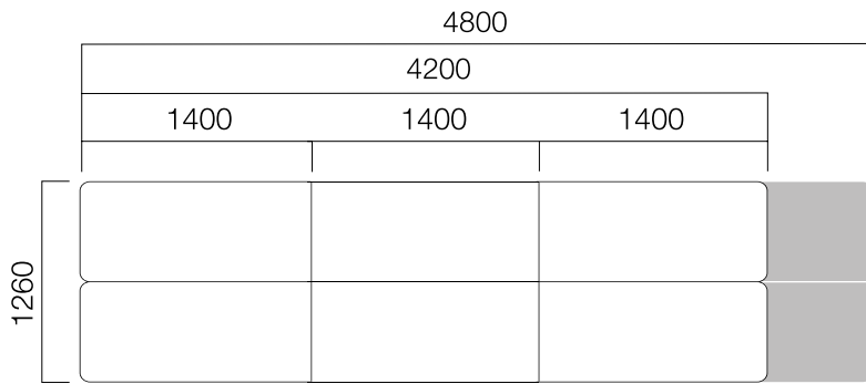
W:126 cm Dörtlü Toplantı Masası
