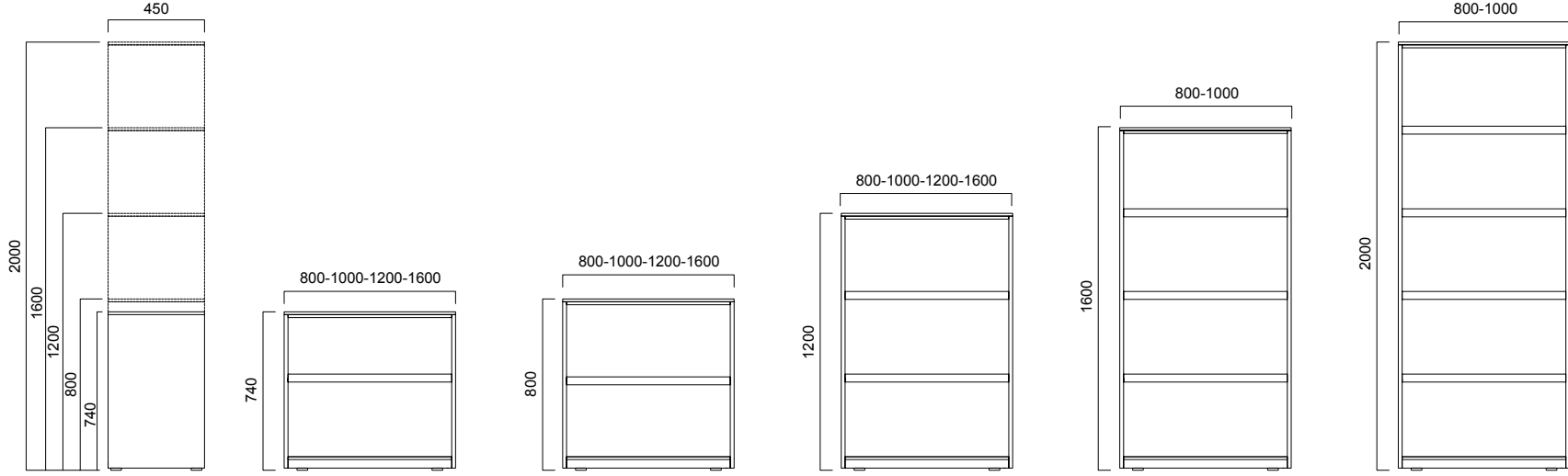
Fe2 Açık Rafli Dolap
