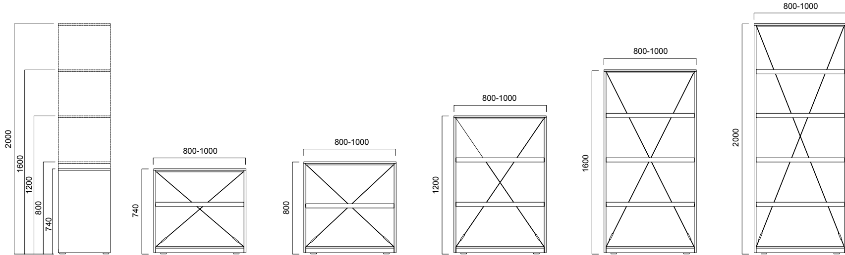
Fe2 Açık Dolap
