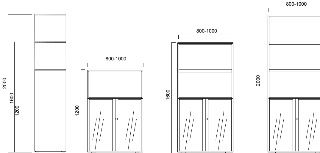
Fe2 Akriik & Cam Kapaklı Açık Rafılı Dolap
