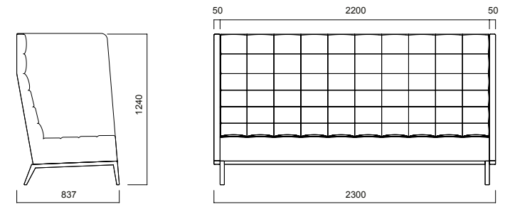
Greta Yüksek Sırtlı Üçlü Koltuk / H:1240
