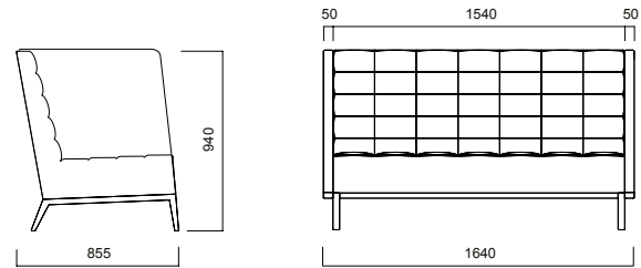
Greta Yüksek Sırtlı İkili Koltuk / H:940
