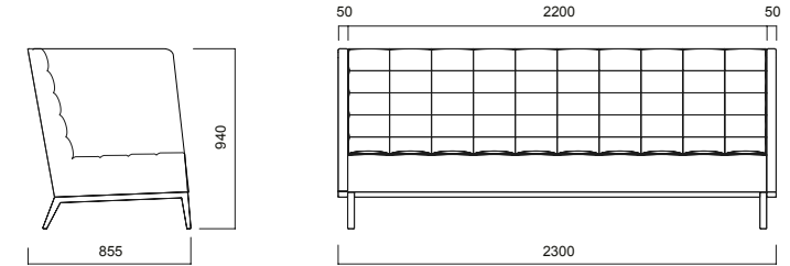
Greta Yüksek Sırtlı Üçlü Koltuk / H:940
