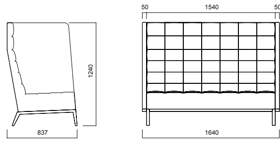
Greta Yüksek Sırtlı İkili Koltuk / H:1240
