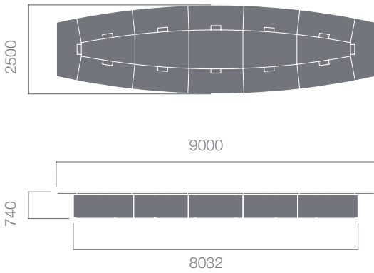
9000mm Toplantı Masası
