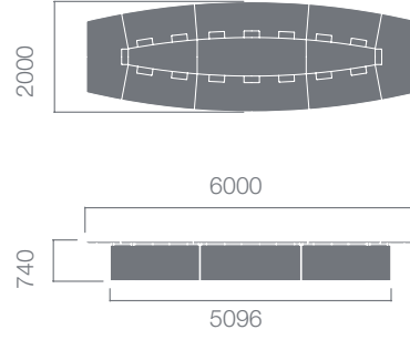
6000mm Toplantı Masası
