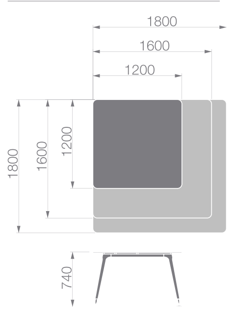
kare 4 ayak
