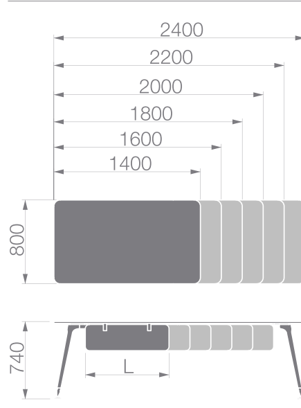
Ön panolar
