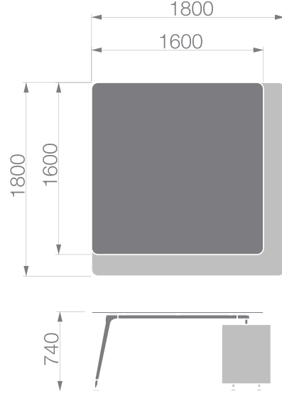
Kare 2 ayak
