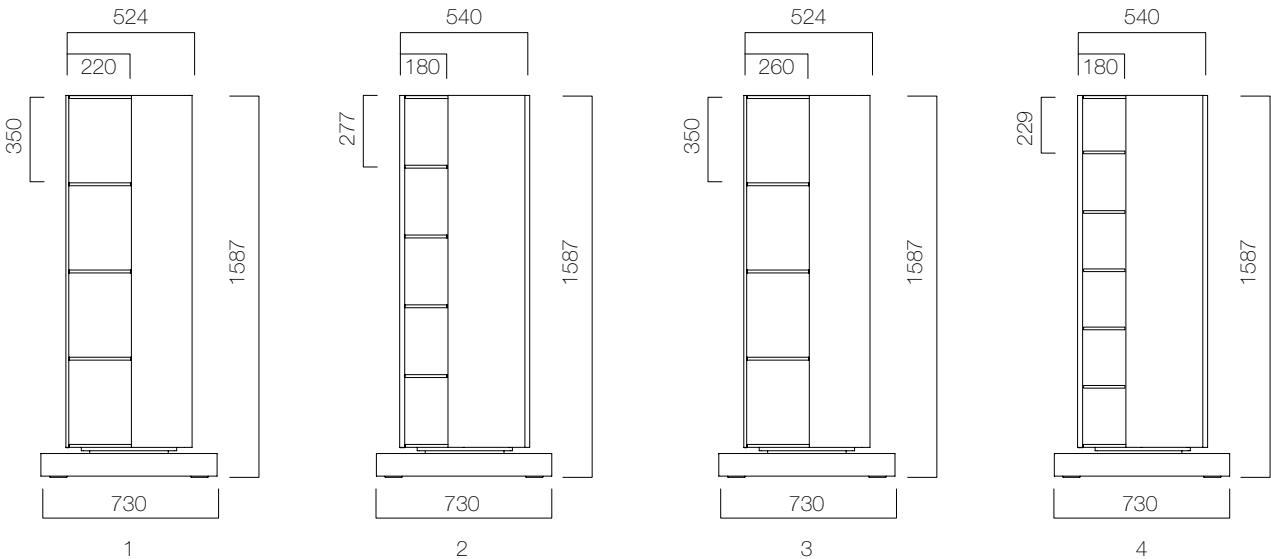
Atlas Single H:158,7 cm
