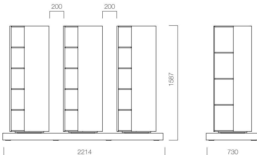
Atlas Triple H:158,7 cm
