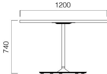
W80X120 H74 Rectangle Table
